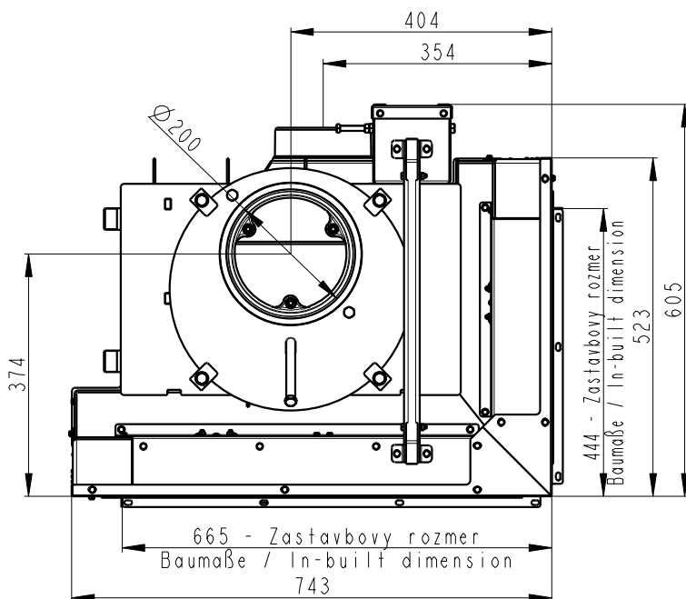
Primarni a sekundarni vzduch Primärluft und Sekundärluft Primary and secondary air
