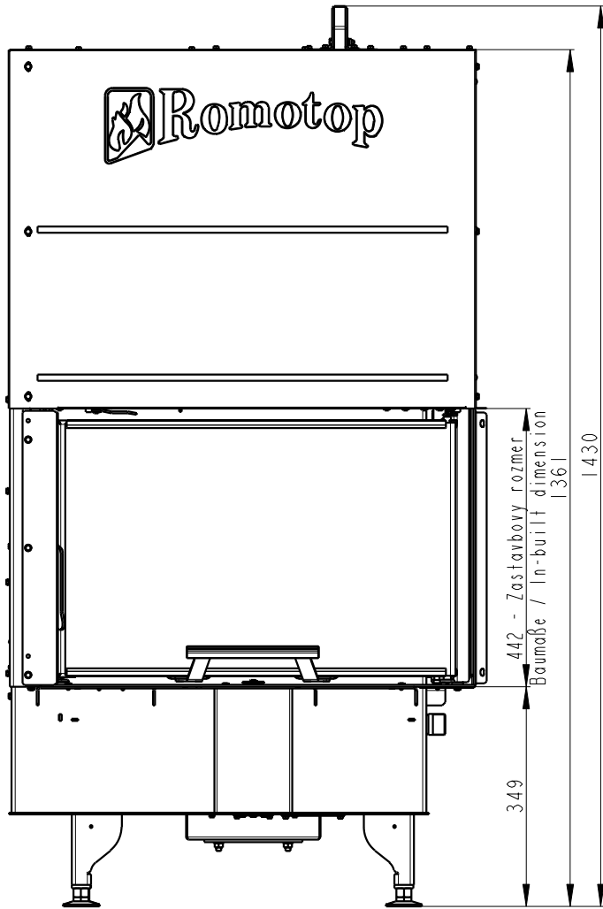
Centralni privod vzduchu Central air inlet Zentralluftzufuhr
